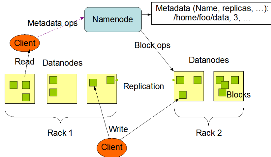
Figura 4: Arquitectura de almacenamiento en Hadoop (HDFS)
